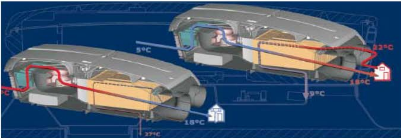
Luchtbehandelaar bestemd voor dakmontage met indirecte verdampingskoeling
