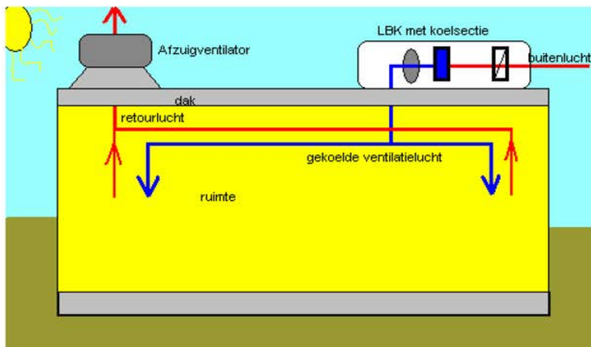
Koeling van ventilatielucht op een bestaand gebouw (zonder warmterugwinning)
